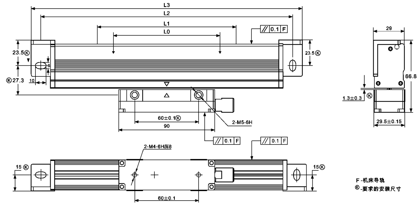
光栅尺 XDGS02 尺寸图
