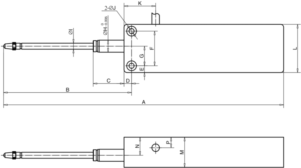
光栅尺 XDGS81 尺寸图
