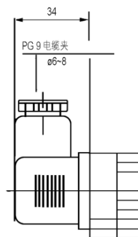
DIN 43650 IP65-ISO4400
