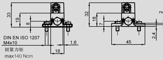
标准型 (Z-45)
