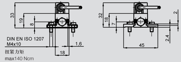
标准型 (Z-45)
