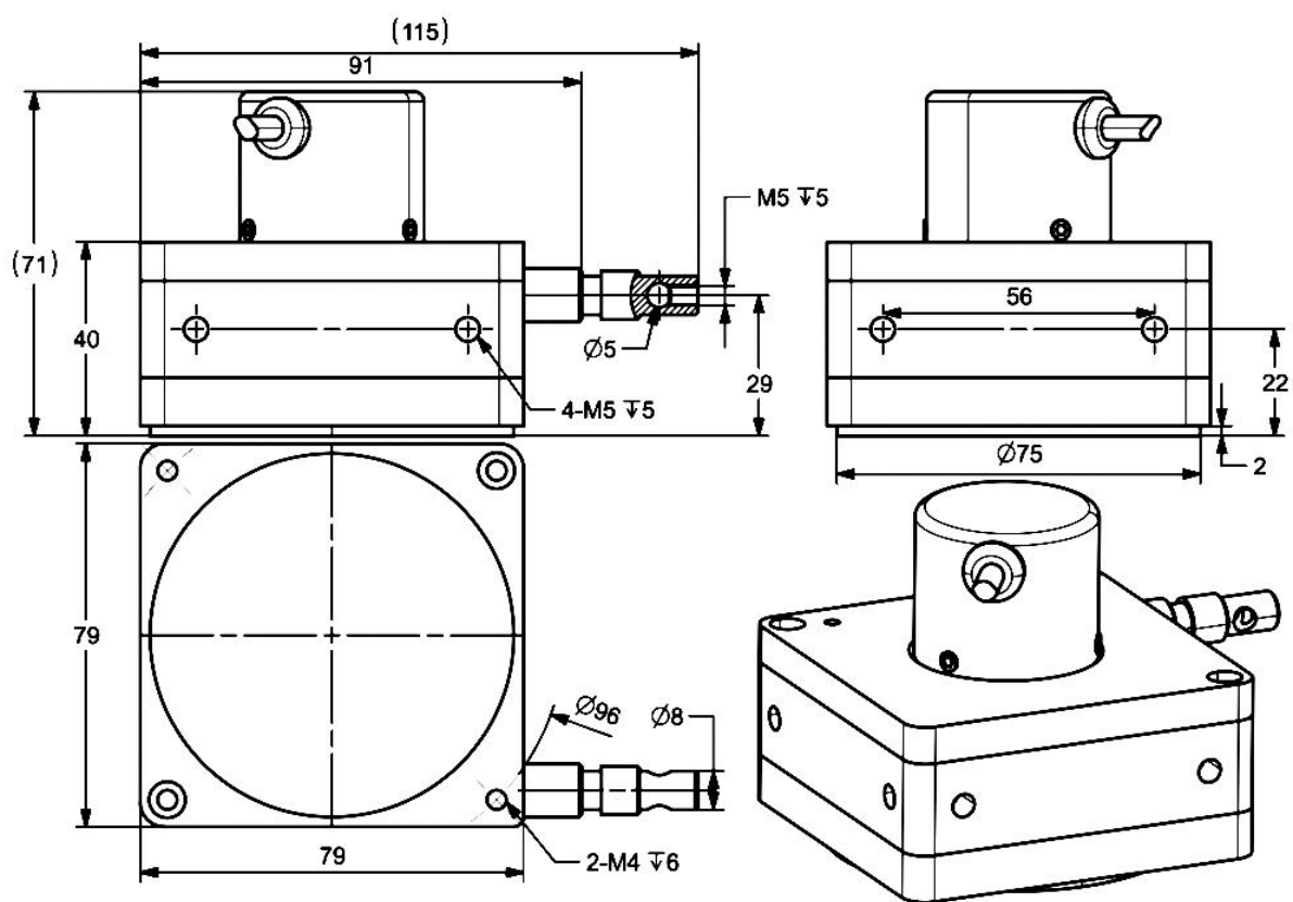
B 款 2m 行程尺寸图
