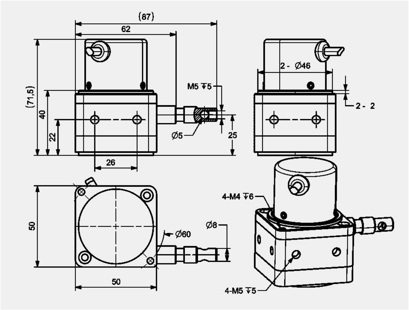
B 款 0.3m&0.5m&1m 行程尺寸图
