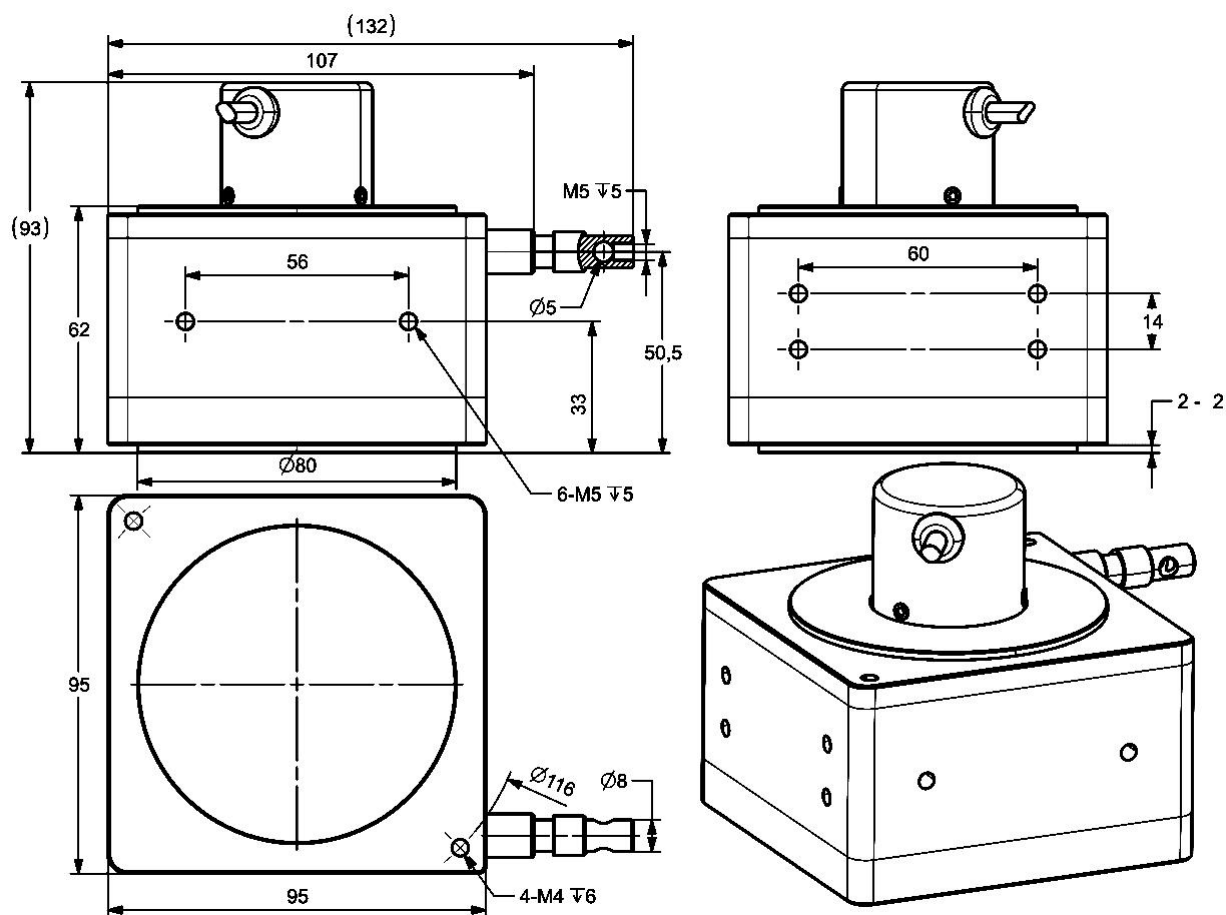
B 款 6m-7m 行程尺寸图
