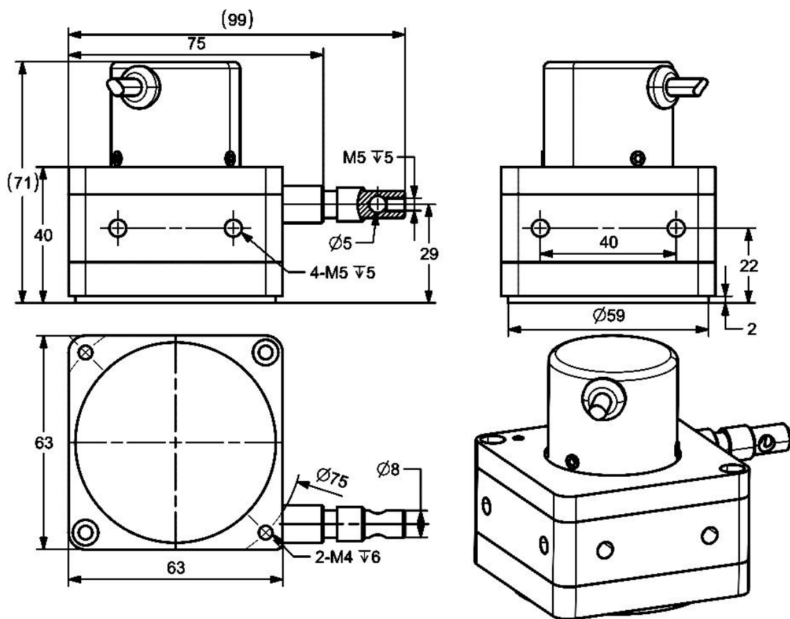
B 款 2m 行程尺寸图
