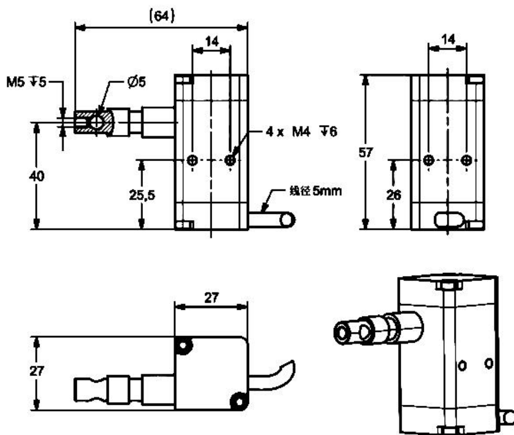
A款 尺寸图
