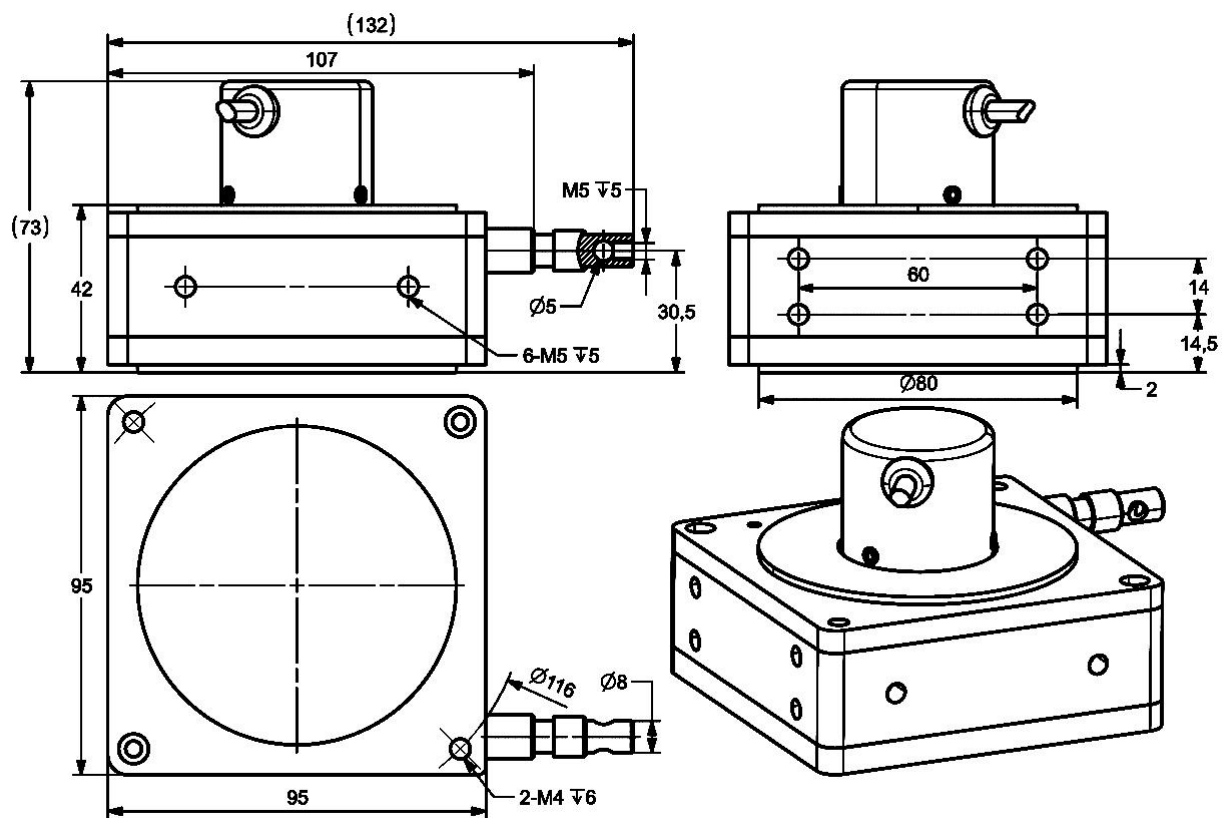
B 款 4m-5m 行程尺寸图
