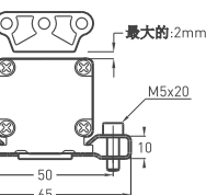
选配固定架
