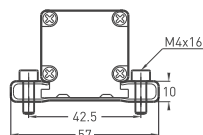
标配固定架
