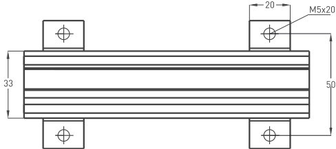
MP2 铝轨
