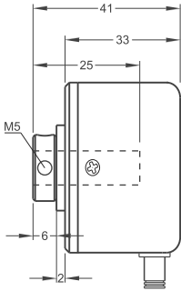
出轴型 / 径向
