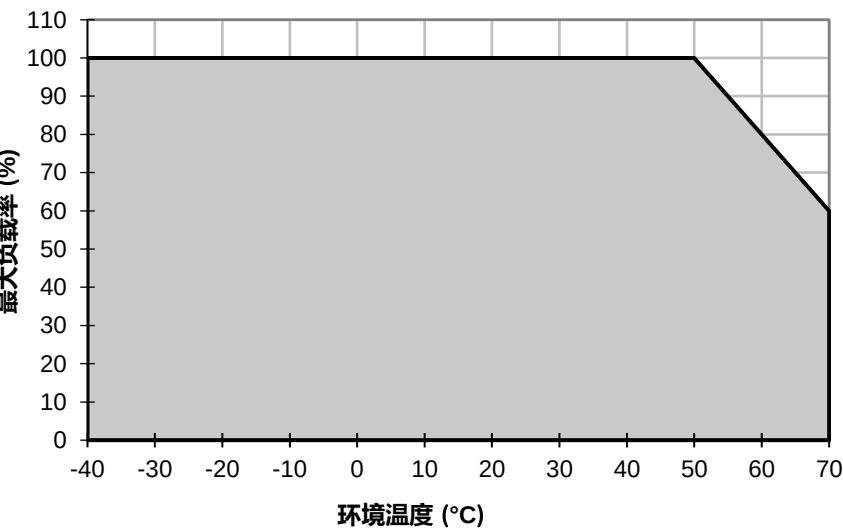
输出负载降额对应环境温度
