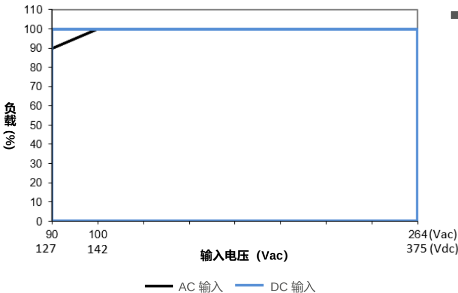
输出负载降额对应输入电压
